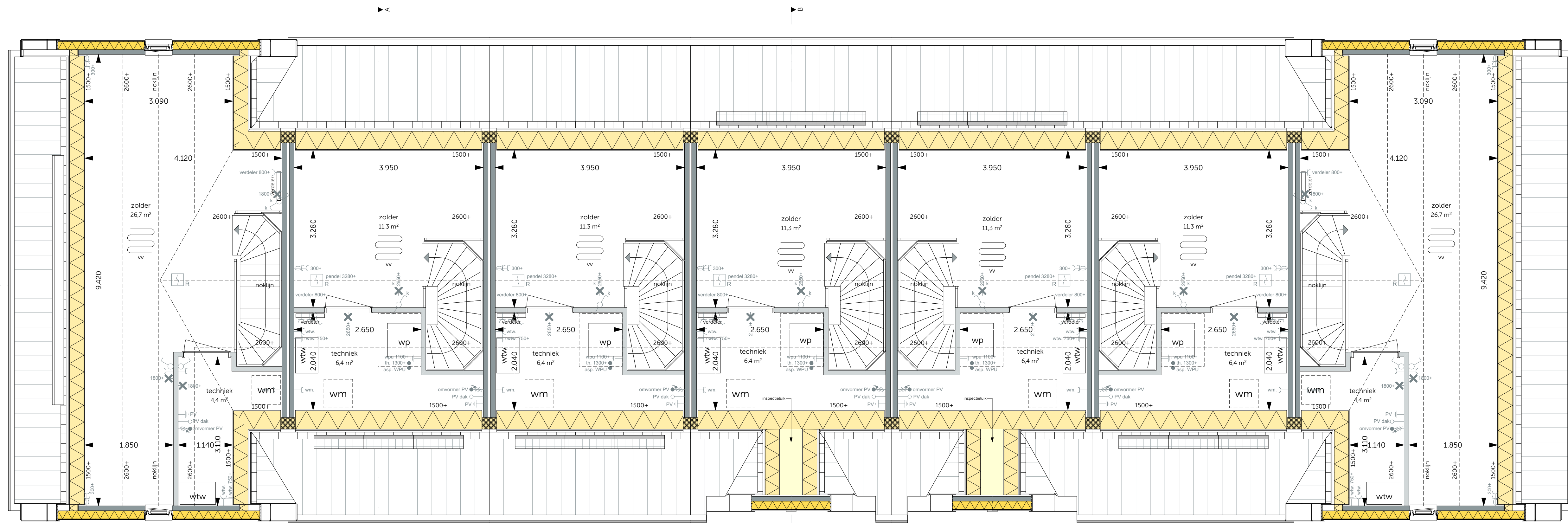
2e verdieping schaal 1:50 BNR 20 5400 Beige BNR 19 type C BNR 18 type C BNR 17 type D BNR 16 type Dsp BNR 15 type Csp BNR 14 5400sp Beige
