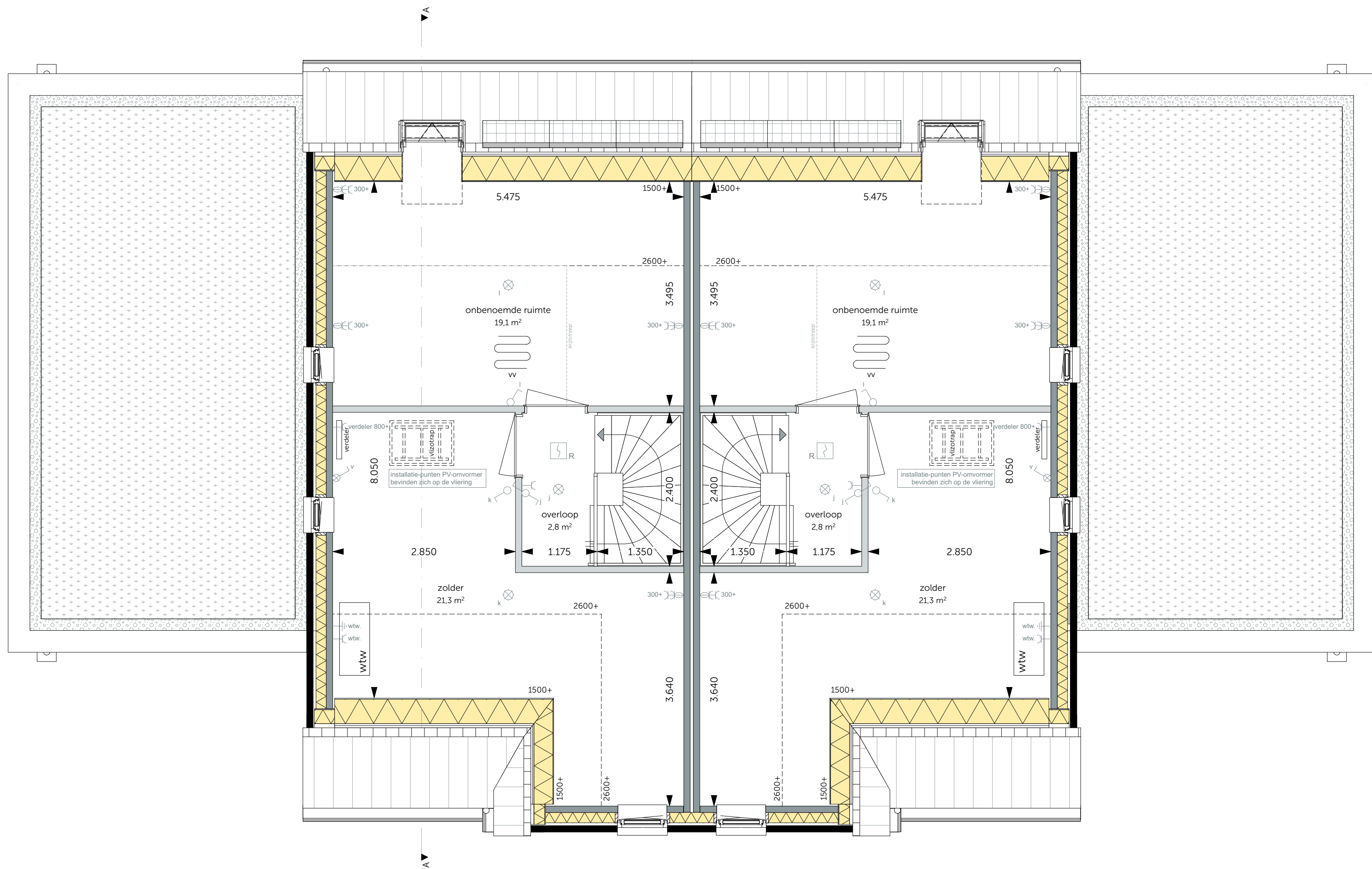
Eerste verdieping schaal 1:50
