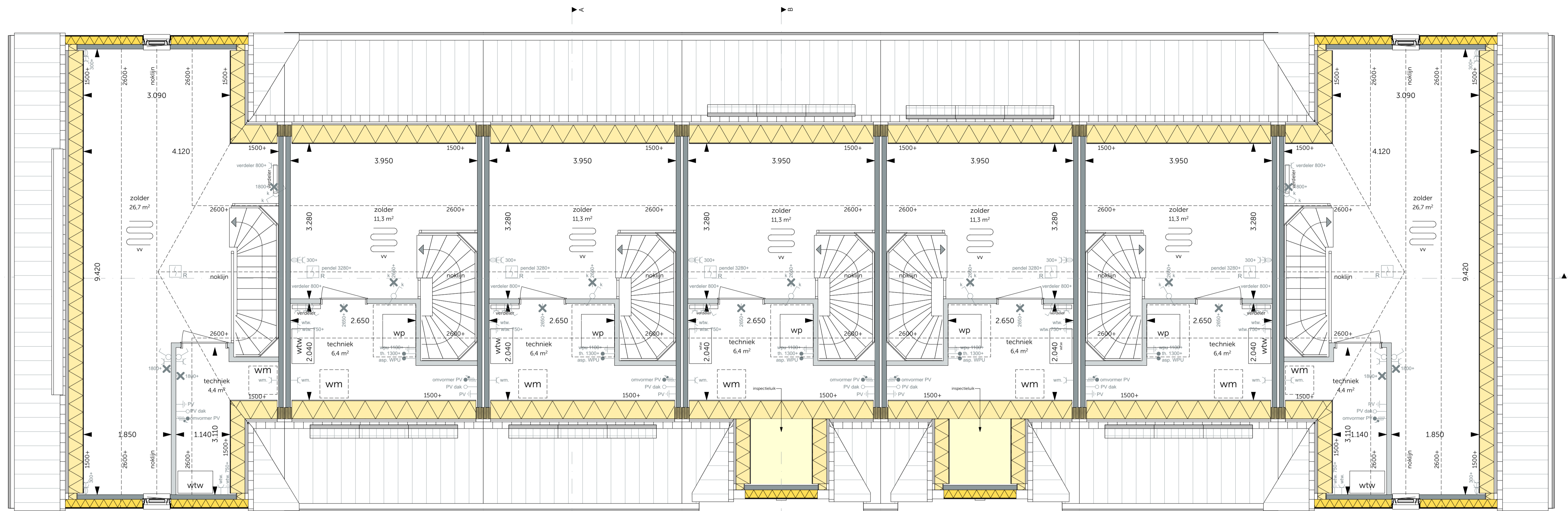
Tweede verdieping schaal 1:50
