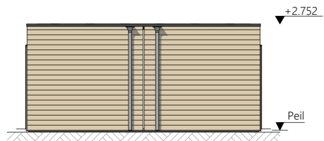
Voorgevel (tuinzijde) schaal 1:100
