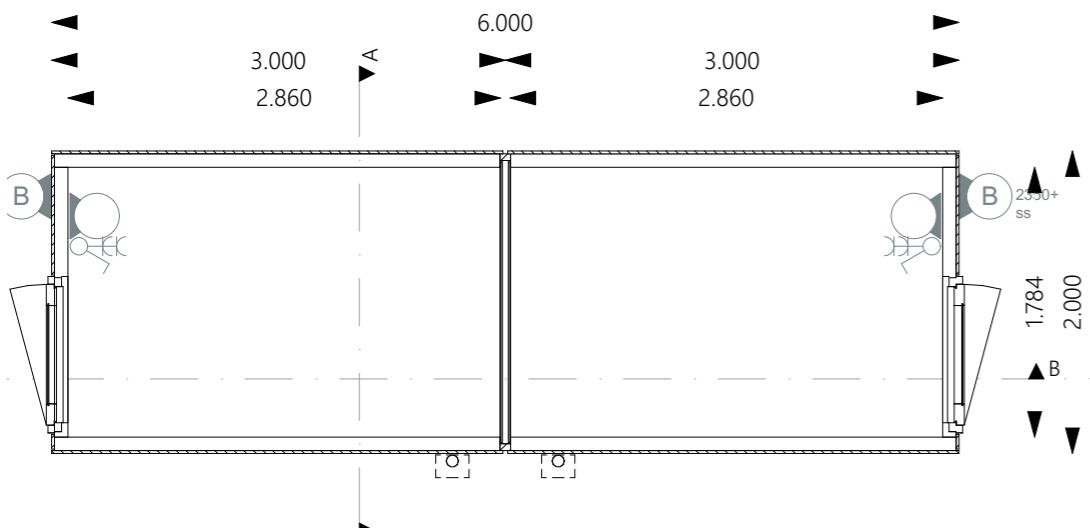
Begane grond schaal 1:50
