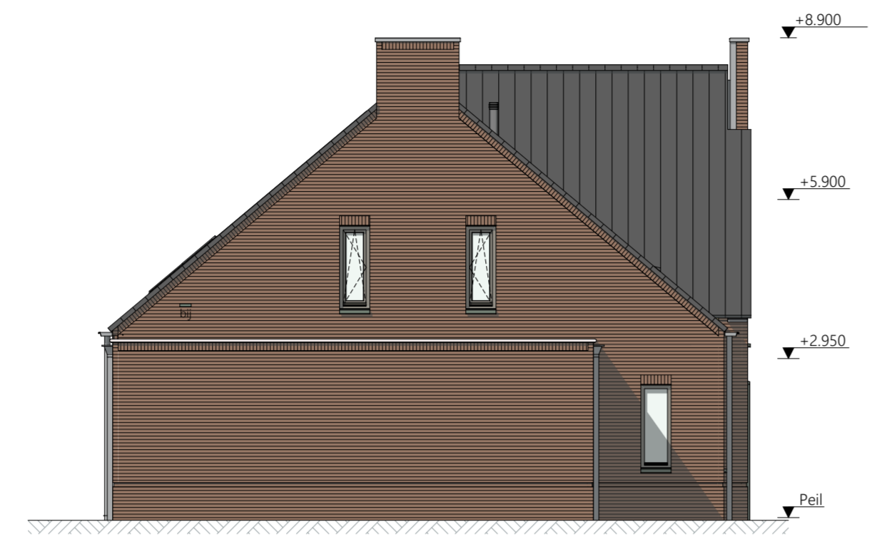
Linkergevel schaal 1:100
